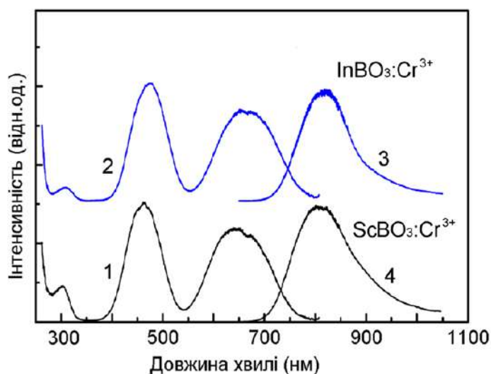
Рис. 1. Спектри збудження (1,2) та люмінесценції (3,4) іонів Cr 3+ у MBO 3 :Cr 3+ (M= Sc, In) при 293 К
