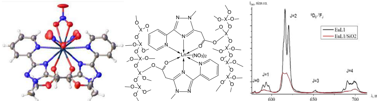
Рис. 1. Кристалічна структура [\text{LaL}_2(\text{NO}_3)_2] , умовна будова люмінесцентного блоку у гібридних матеріалах (Ln = Nd(III), Eu(III), Tb(III), X = Si(IV), Ti(IV), Al(III)), порівняння спектрів люмінесценції комплексу європію та гібридного матеріалу на його основі
