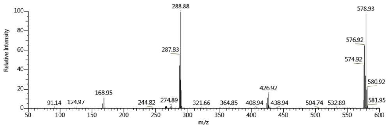
Рис. 1. ESI(-)-мас-спектр водно-метанольного розчину [Ge(H 3 Gal) 2 (H 2 Gal)]·2H 2 O
