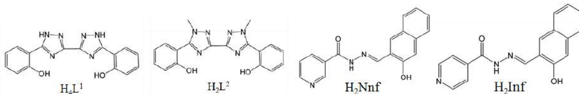
Рис. 1. Схематична будова використаних основ Шиффа
